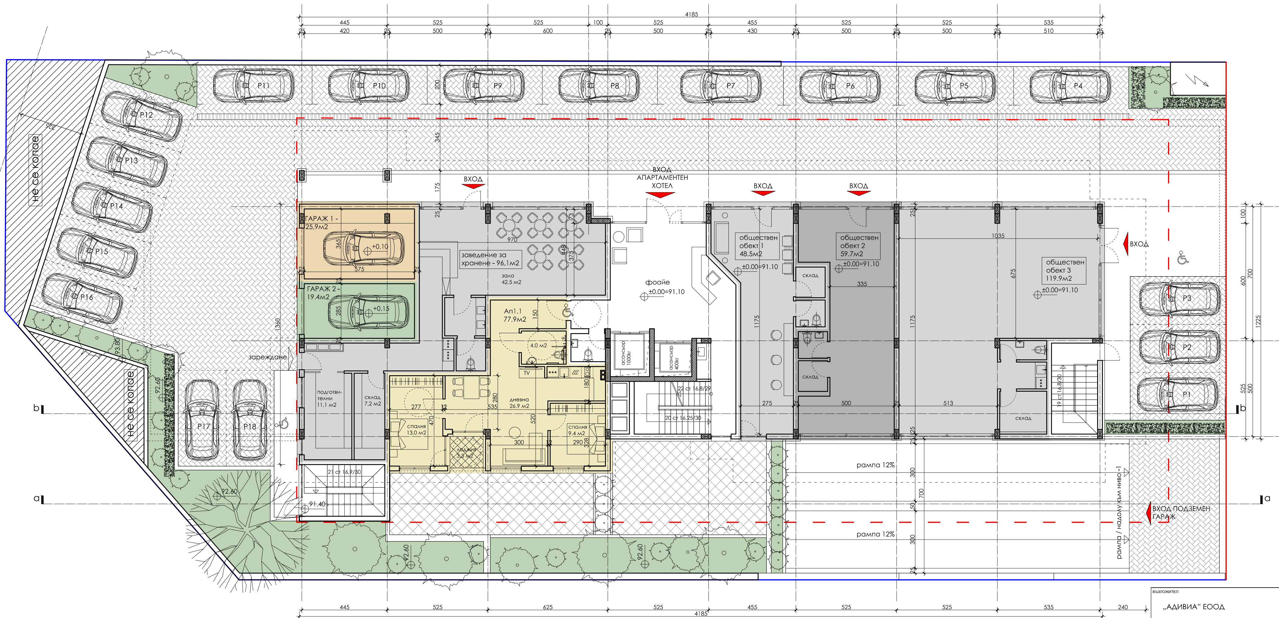
РАЗПРЕДЕЛЕНИЕ 1етаж - 560.0м2
