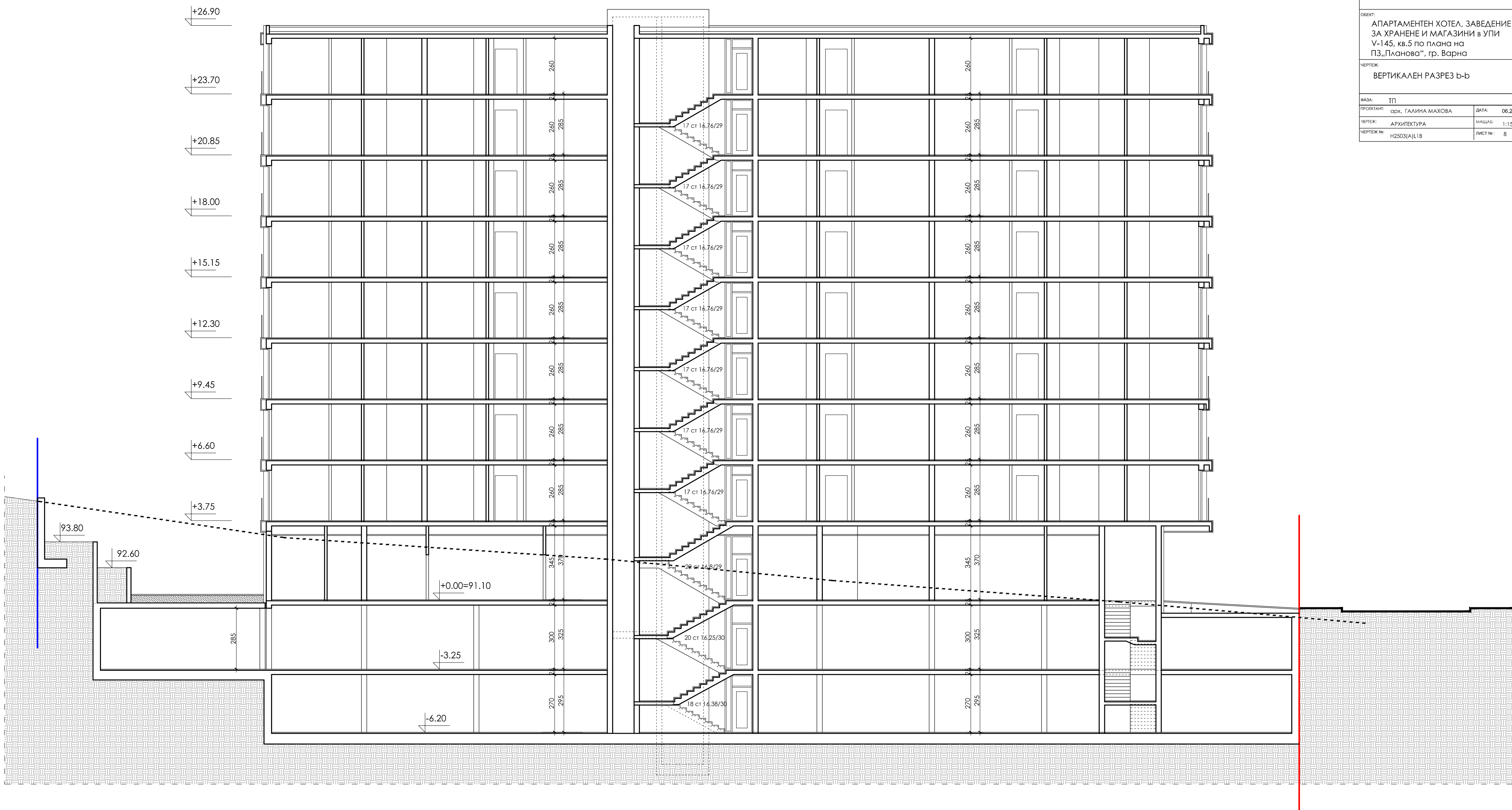
ВЕРТИКАЛЕН РАЗРЕЗ b-b
